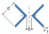
2 (VVLM) Cantoneiras laminadas opostas pelos vértices
