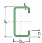
U formado a frio enrijecido
