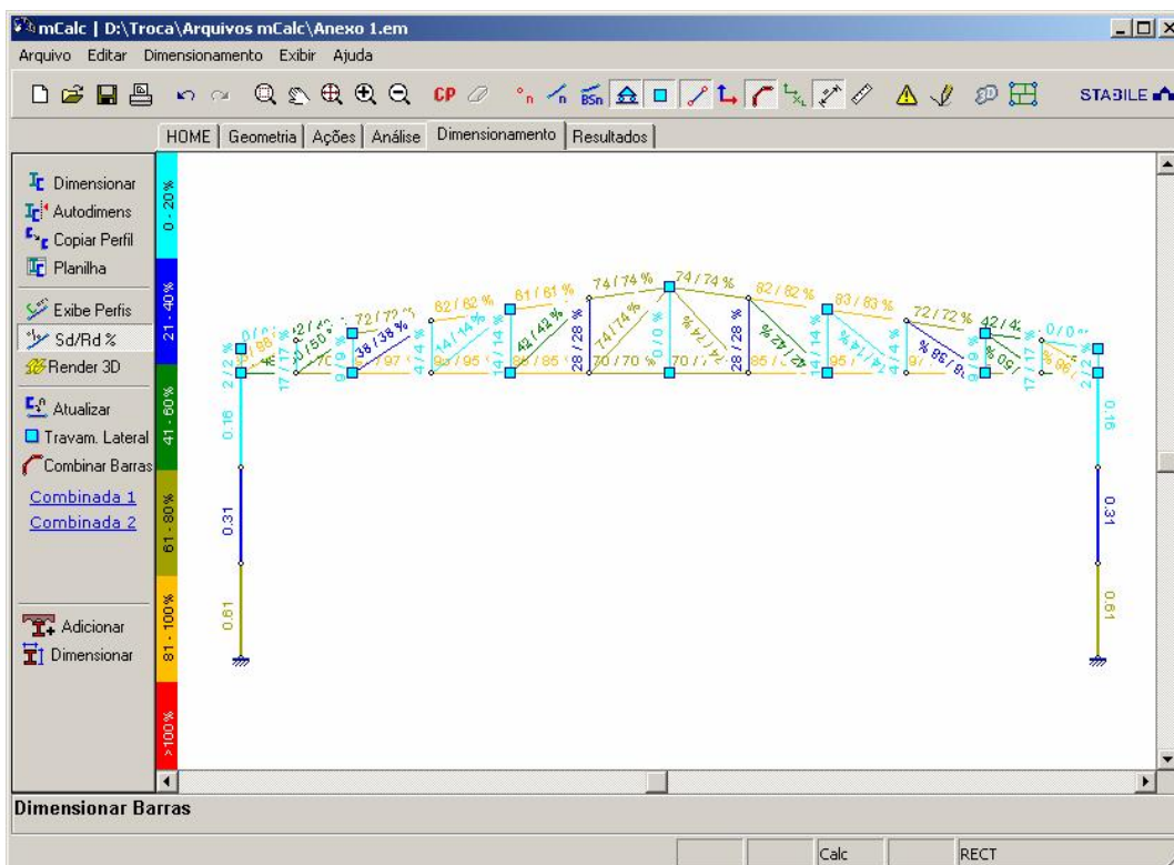
Estrutura dimensionada
