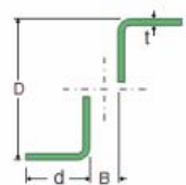
2 Cantoneiras (FF) em Z
