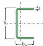
U formado a frio
