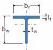
Tee laminado-metade do açominas (TW)
