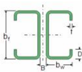
I (FF) enrijecido
