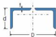
2 (LLLM) Cantoneiras laminadas opostas pelas mesas
