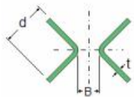
2 Cantoneiras (FF) opostas pelos vértices
