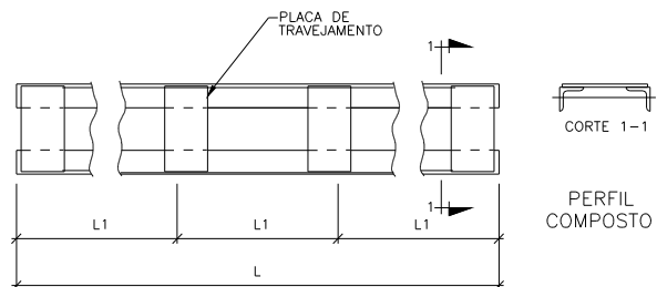
Perfil Composto
