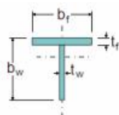
T soldado (TS)
