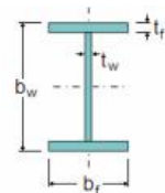
I viga soldada (VS)
